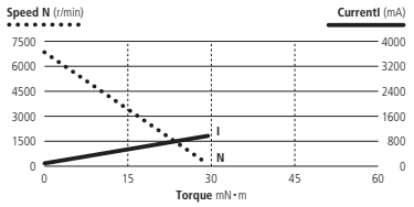
EN35 M 24V
