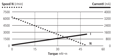
EN35 L 24V
